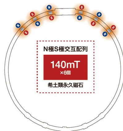
磁石配置図
