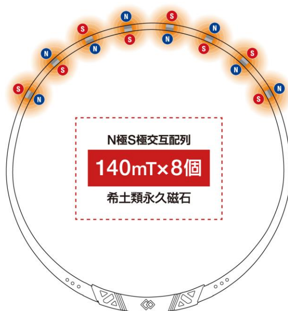
磁石配置図
